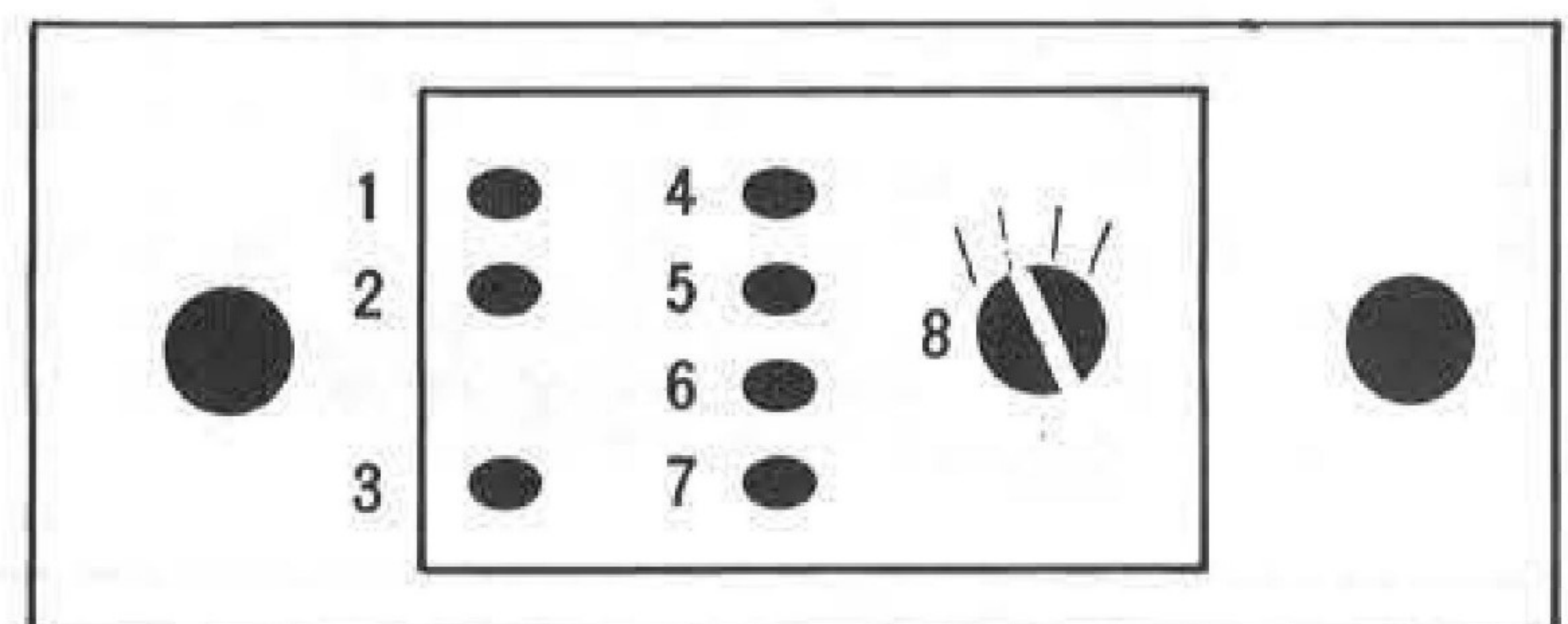
盤面略図
