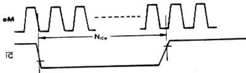
Fig. A-2 Reset Timing
