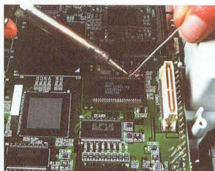
▲ Jetzt wird es ernst, Zeit zum Löten! Verbindet nun äußerst vorsichtig die vier in Abbildung A (unten Mitte!!!) markierten Punkte mit dem BIOS-Baustein.
