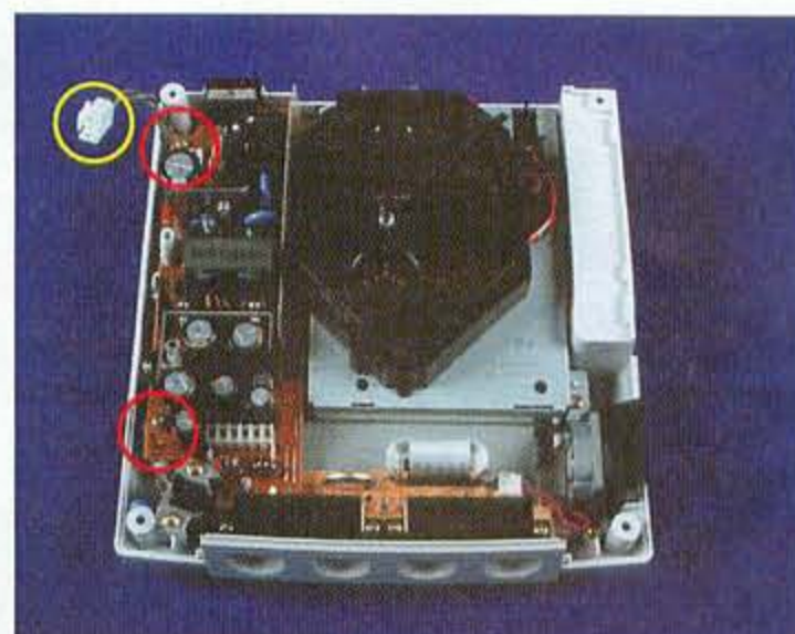
▲ Dreht die Konsole wieder um, so dass die vier Controller-Ports zu euch zeigen. Löst zuerst den weißen Netzstecker (gelber Kreis) und entfernt dann behutsam die zwei Schrauben (rot), die das Netzteil befestigen.
