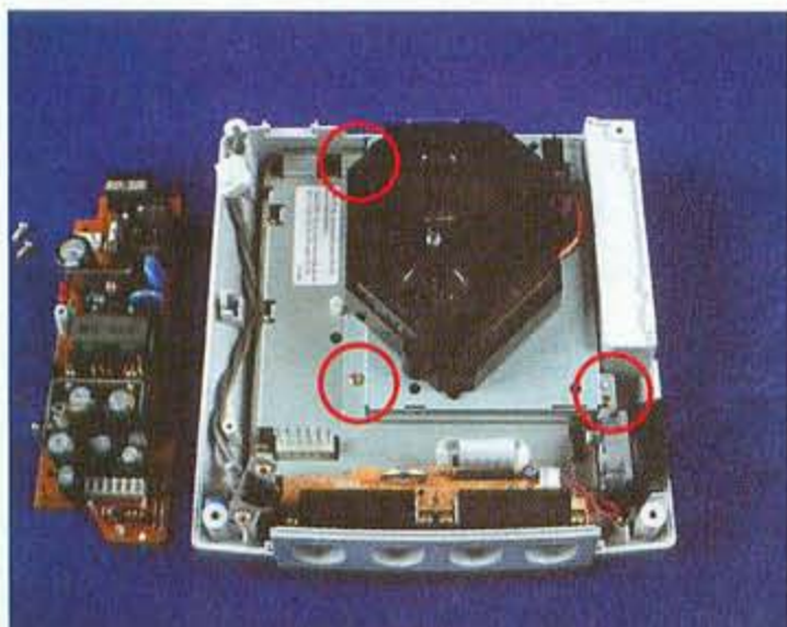
▲ Nachdem das Netzteil und der darunter liegende Plastenschutz entfernt wurden, löst ihr die drei Schrauben, mit denen das GD-ROM Laufwerk montiert ist. Nachfolgend legt ihr dieses ganz sorgsam zur Seite.
