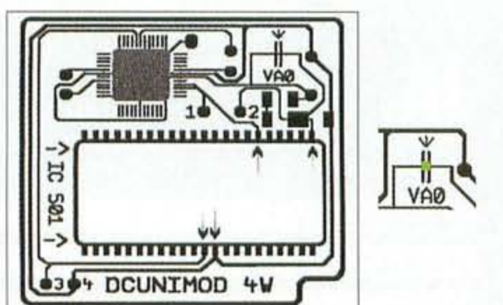
▲ Hier seht ihr nochmal an welchen Stellen (oben mit schwarzen Pfeilen markiert) genau gelötet werden muss. ACHTUNG: Bei älteren DC, die in der Nähe der Padanschlüsse mit VA0 gekennzeichnet sind, muss die mit einem Pfeil markierte Leiterbahn (in der kl. Abb. grün dargestellt) mit einem scharfen Messer durchtrennen. Ansonsten keine anderen Leiterbahnen durchtrennen!!! Bei VA1 Boards nichts ändern!!!
