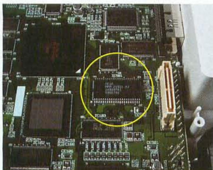
▲ Hier seht ihr den BIOS-Baustein noch einmal in einer Nahaufnahme. Er müsste die Bezeichnung SEGA MPR-XXXXXX tragen (X können in diesem Fall irgendwelche Zahlen sein).
