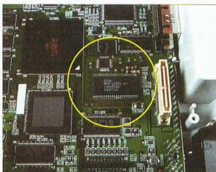
▲ Positioniert nun den MOD-Chip so, dass sich die ausgesägte Ecke rechts neben der Aufschrift DCUNIMOD 4W am unteren rechten BIOS-Fuss befindet.
