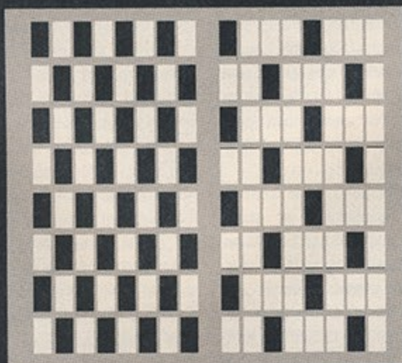
• 50 per cent and 25 per cent dithering patterns.
