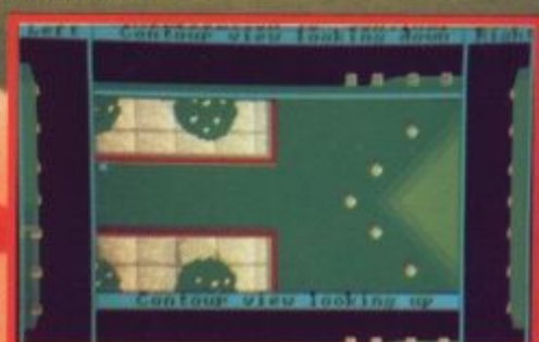
ATARI ST
