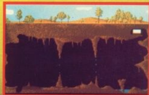
AMIGA
