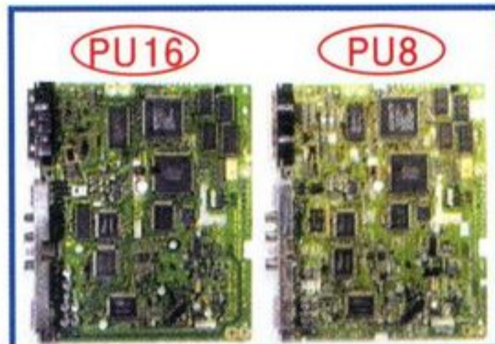
왼쪽에 있는 기관이 화이트 플스의 기관인 PU-16이다. 플스 3500의 기관인 PU-8(오른쪽)과 거의 비슷하다
