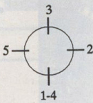
Earth
