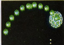
Pluto
