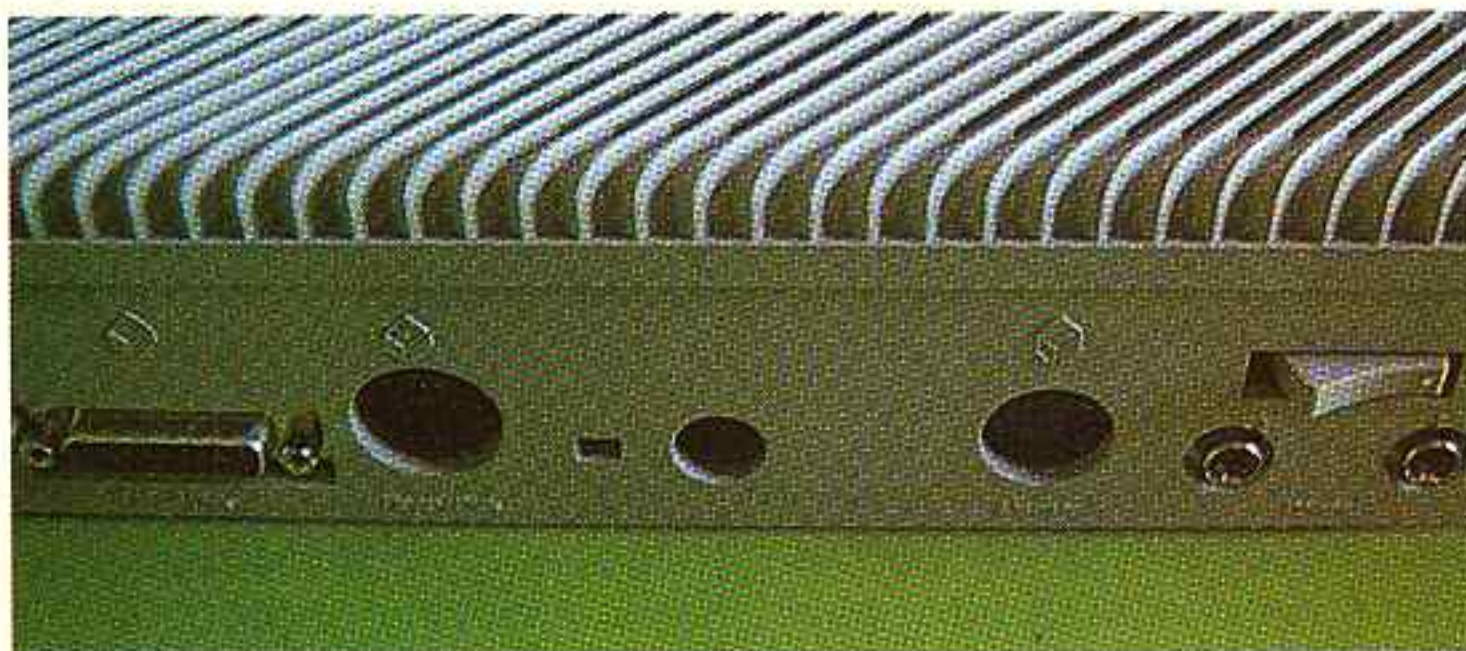
La face arrière du STE dévoile de nouveaux connecteurs. Des sorties son de type Cinch et un orifice Genlock font en effet leur apparition.
