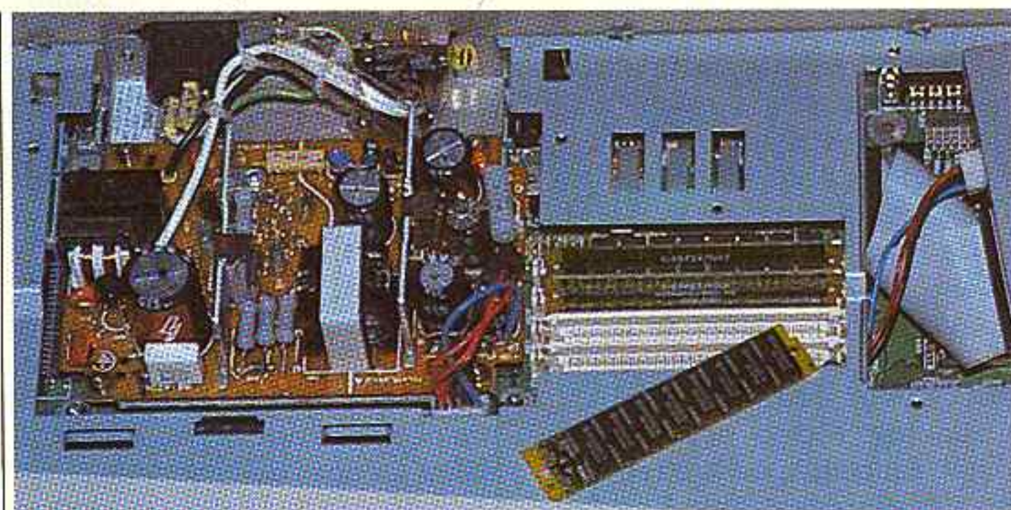
Innovation marquante du STE: il permet d'étendre assez facilement la mémoire centrale de la machine jusqu'à 4 Mo de RAM.
