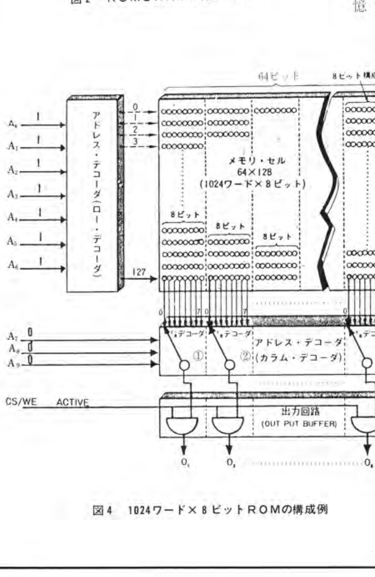
図4 1024ワード×8ビットROMの構成例
