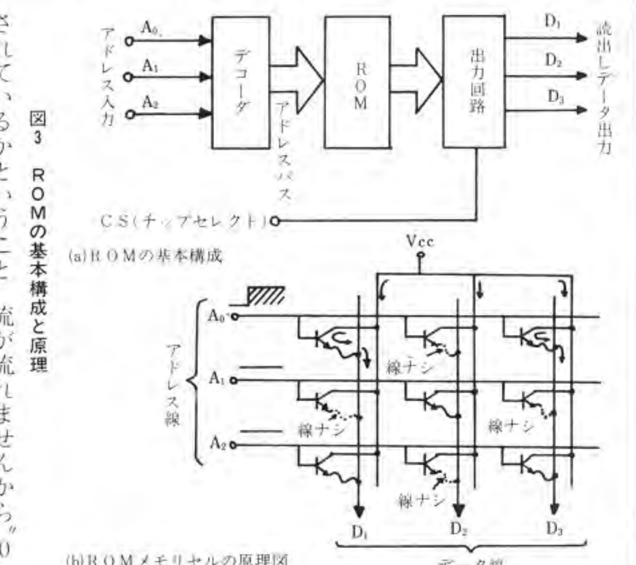
図3 ROMの基本構成と原理
