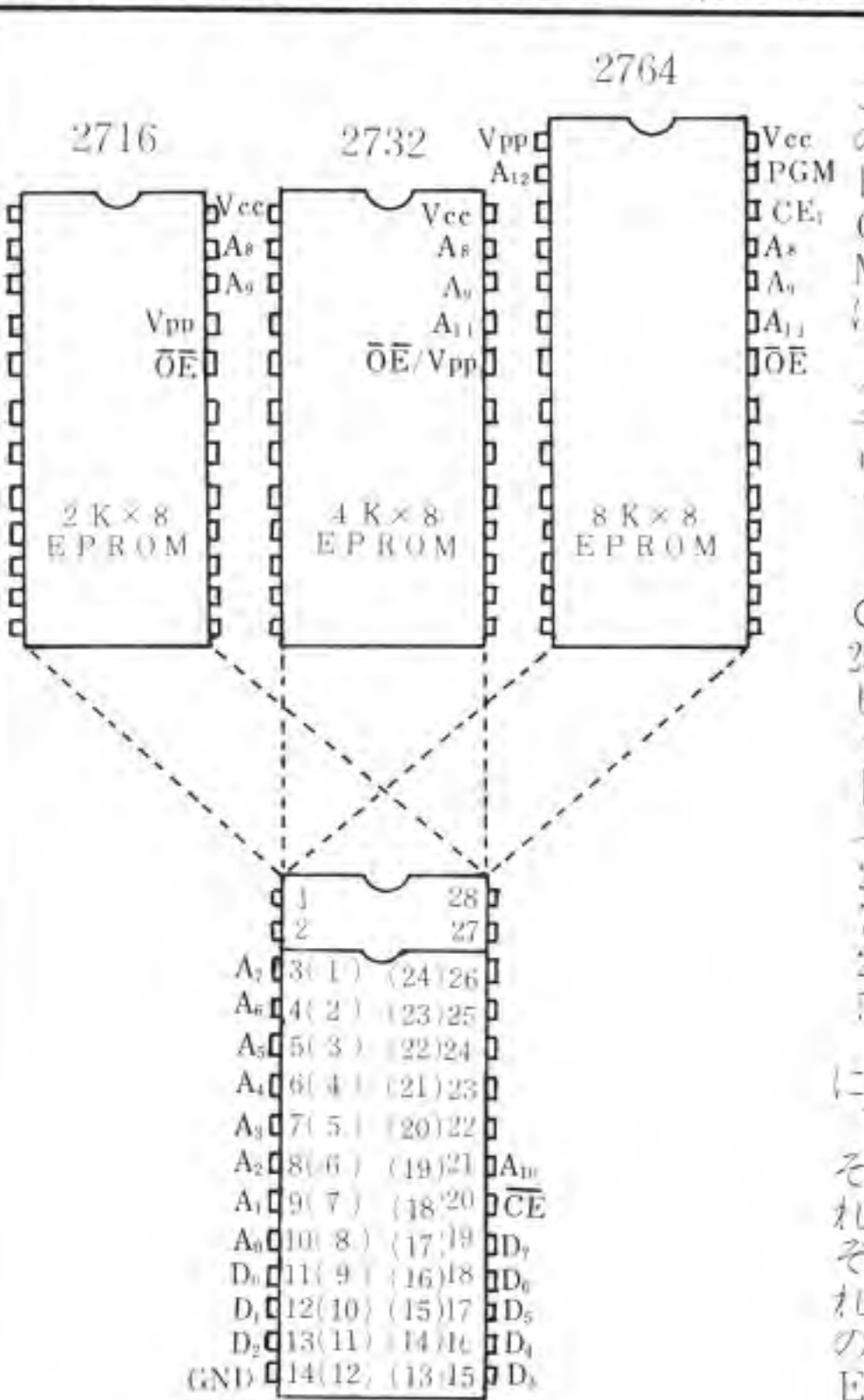
図5 3種類のEPROMのピン配置の違い
