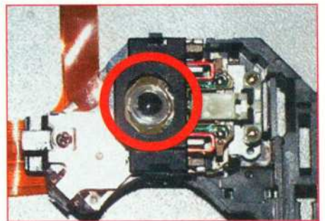
Bitte Vorsicht: Die Laserlinse reinigt Ihr mit einem Wattestäbchen und etwas reinem Alkohol (kein Bier oder Wiskey).
